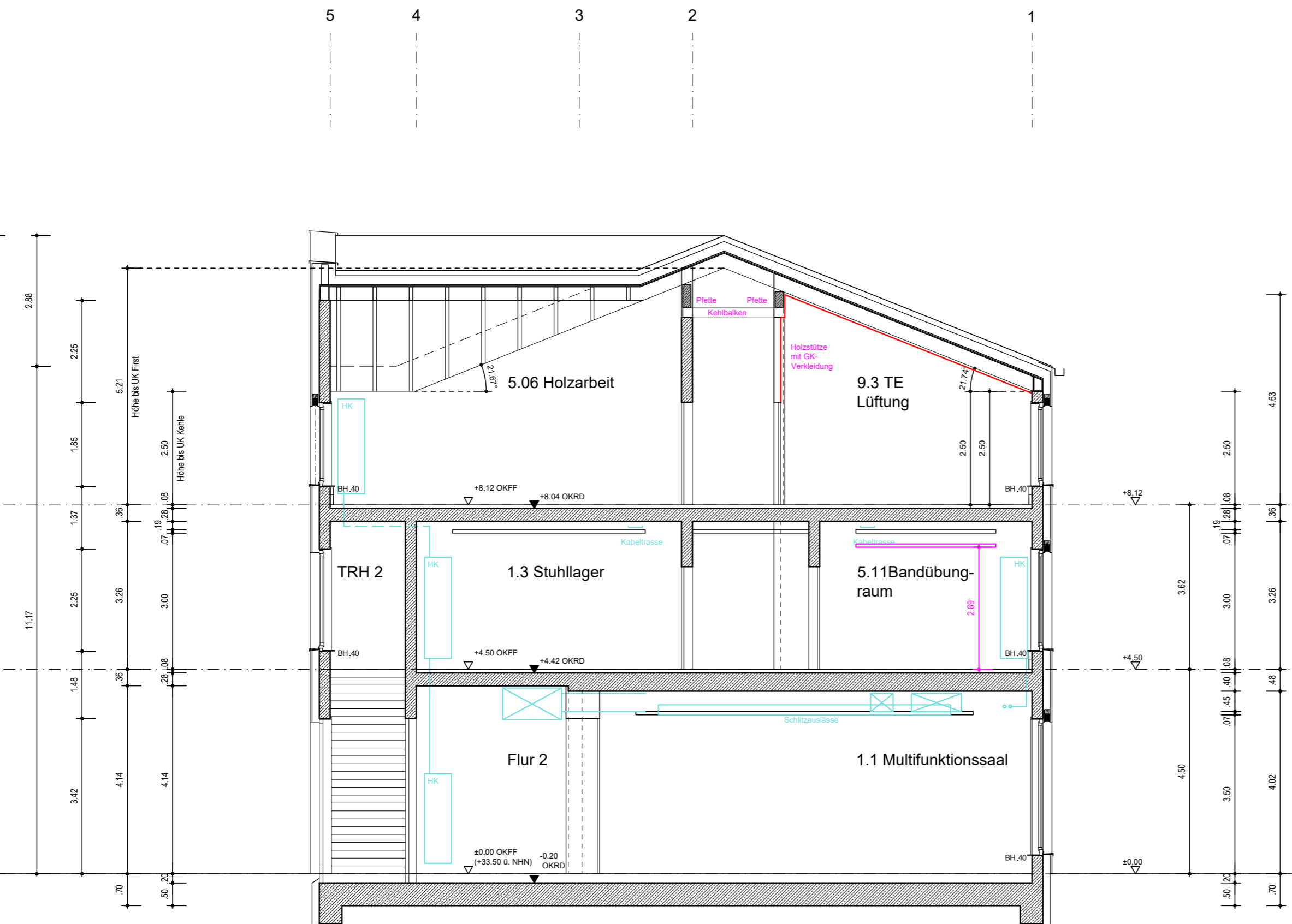
Gebäudeschnitt
